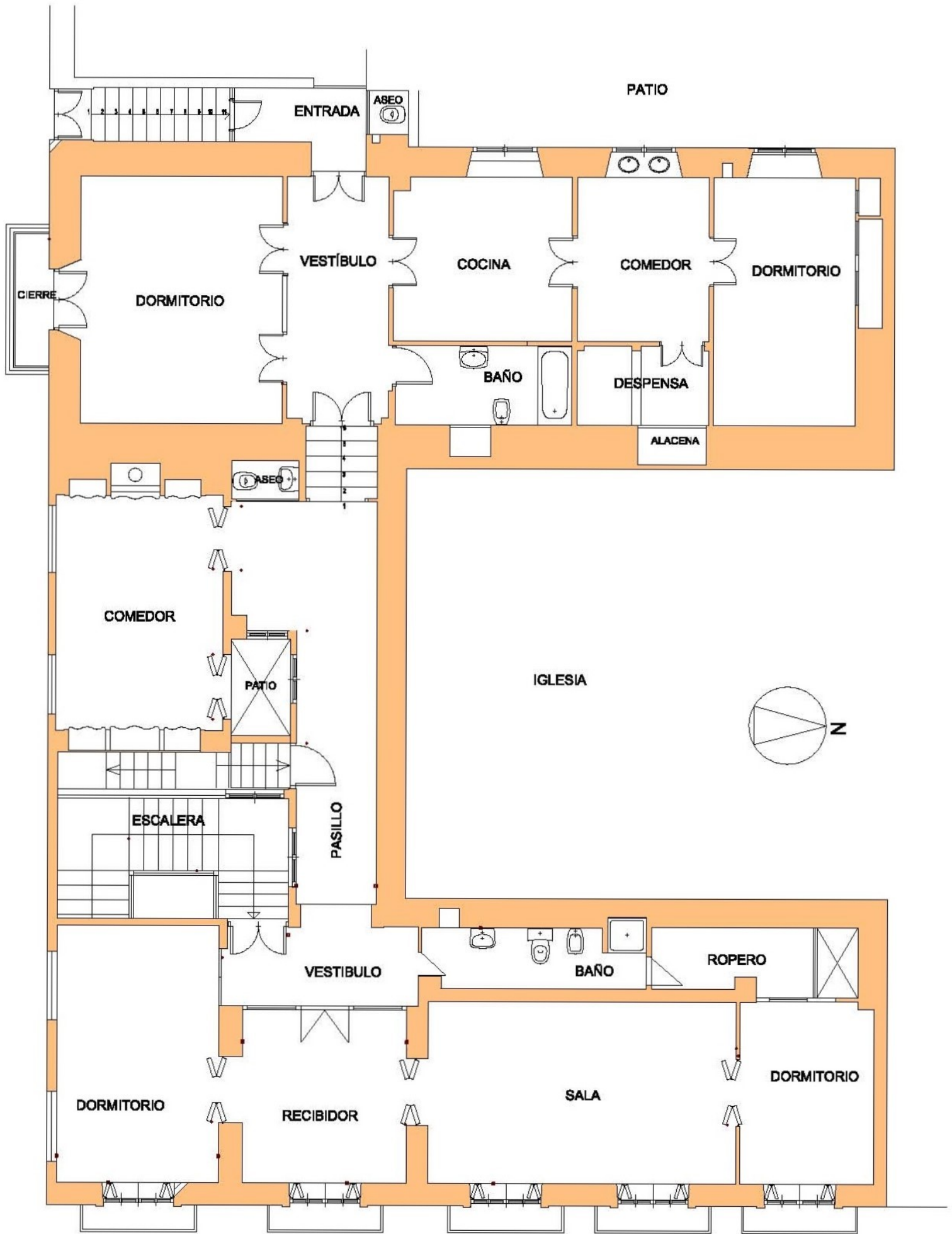
PLANTA PRINCIPAL
