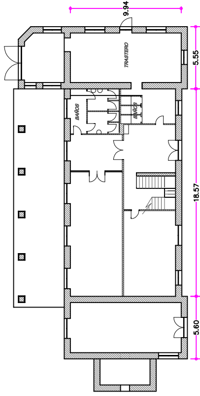
Planta baja (443 m2.)
