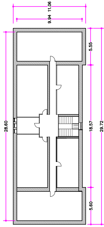
Bajo cubierta (319 m2.)
