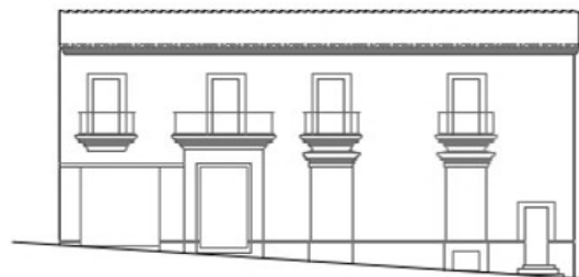
ALZADO A CALLE MESONES
